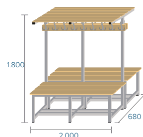
BANC-3-2000-DC 61kg · 0,64m 3 · 18 ↓
