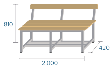
BANC-4-2000 20,5kg · 0,68m 3
