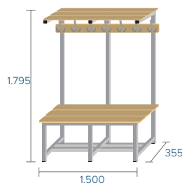
BANC-3-1500 28,5kg · 0,36m 3 · 7 ↓
