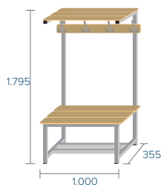
BANC-3-1000 21,5kg · 0,28m 3 · 4 ↓
