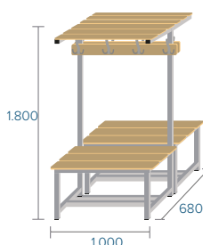
BANC-3-1000-DC 37kg · 0,48m 3 · 8 ↓
