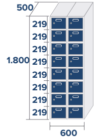
ECO-30/2 COD: 83822 48,4kg, 0,54m 3
