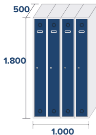
ECO-25/4 COD:82504 50,3kg,0,9m 3
