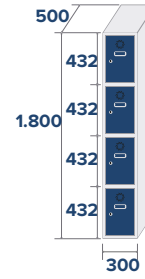
ECO-30/1 COD: 83021 22,3kg 0,27m 3
