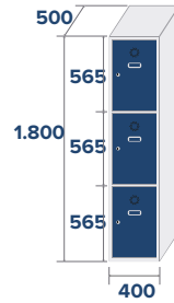
ECO-40/1 COD: 84031 24,2kg 0,36m 3
