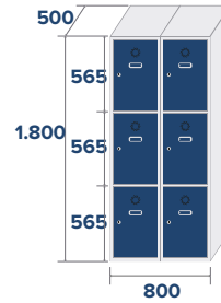
ECO-40/2 COD: 84032 42,4kg 0,72m 3
