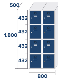
ECO-40/2 COD: 84022 45,4kg 0,72m 3
