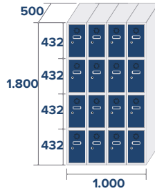
ECO-25/4 COD: 82524 65,2kg 0,9m 3
