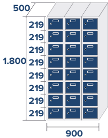
ECO-30/3 COD: 83823 70,1kg, 0,81m 3
