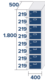
ECO-40/1 COD: 84821 30,9kg, 0,36m 3
