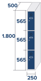
ECO-25/1 COD: 82531 19,9kg 0,22m 3
