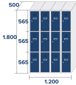
ECO-30/4 COD: 83034 66,8kg 1,08m 3
