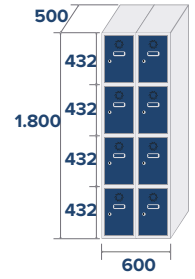
ECO-30/2 COD: 83022 38,6kg 0,54m 3
