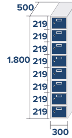
ECO-30/1 COD: 83821 26,7kg, 0,27m 3
