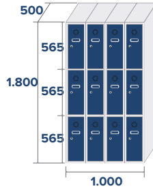
ECO-25/4 COD: 82534 61,6kg 0,9m 3
