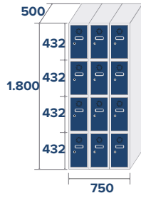
ECO-25/3 COD: 82523 50,4kg 0,67m 3
