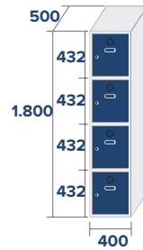
ECO-40/1 COD: 84021 25,7kg 0,36m 3
