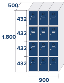
ECO-30/3 COD: 83023 54,9kg 0,81m 3
