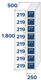
ECO-25/1 COD: 82581 24,4kg, 0,22m 3
