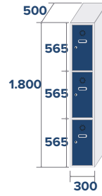
ECO-30/1 COD: 83031 21,2kg 0,27m 3
