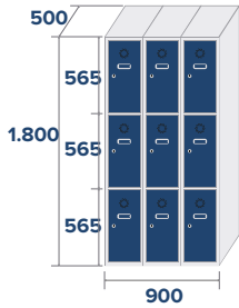
ECO-30/3 COD: 83033 51,6kg 0,81m 3
